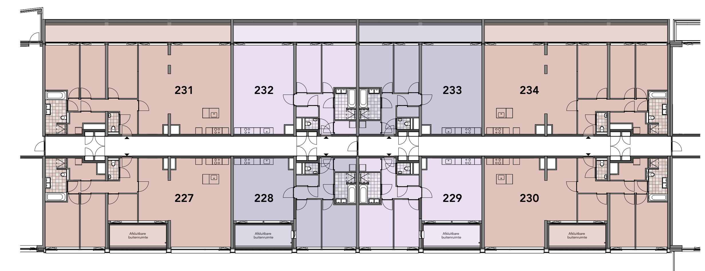
5e verdieping
