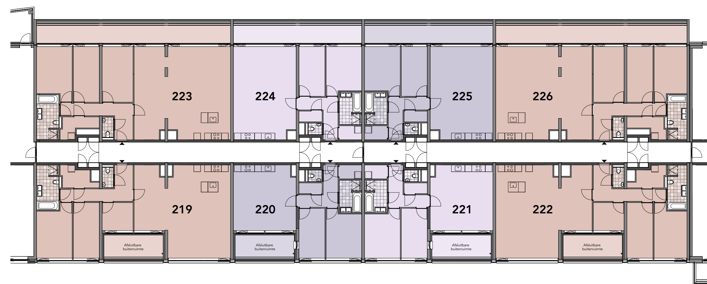
4e verdieping
