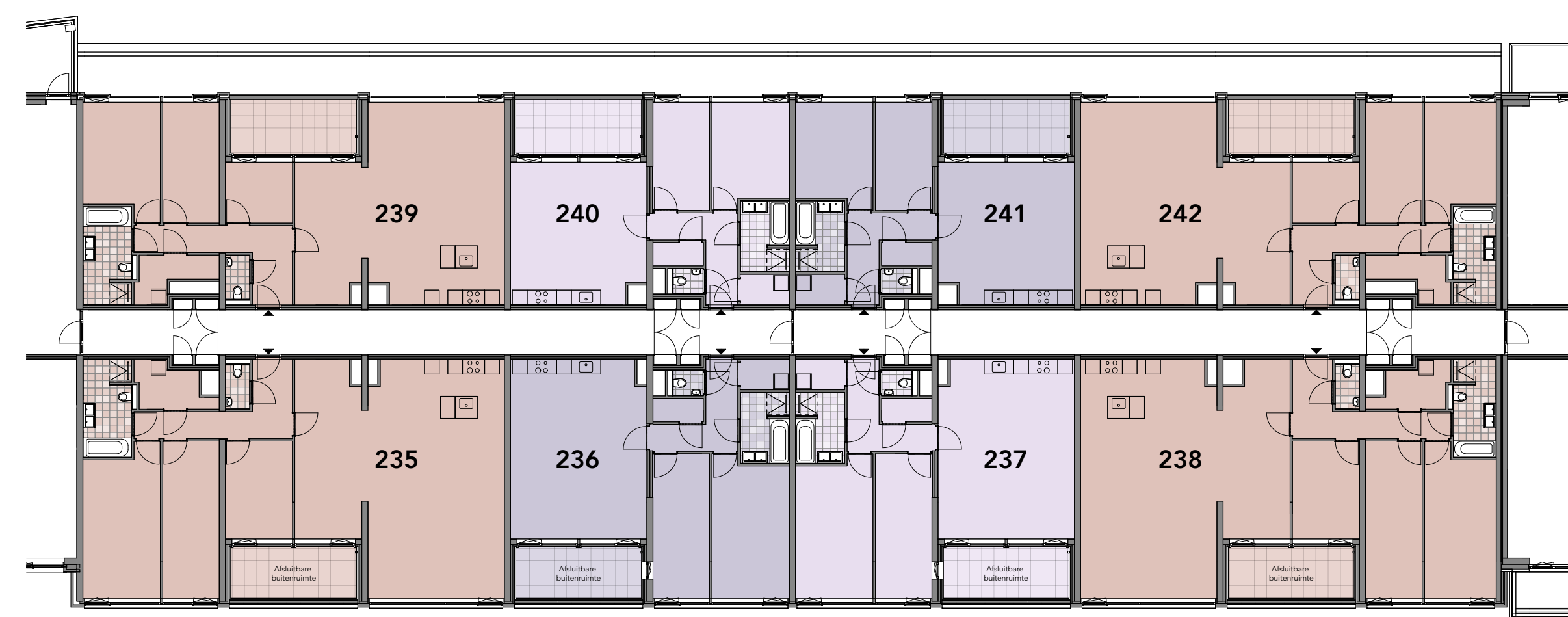
6e verdieping
