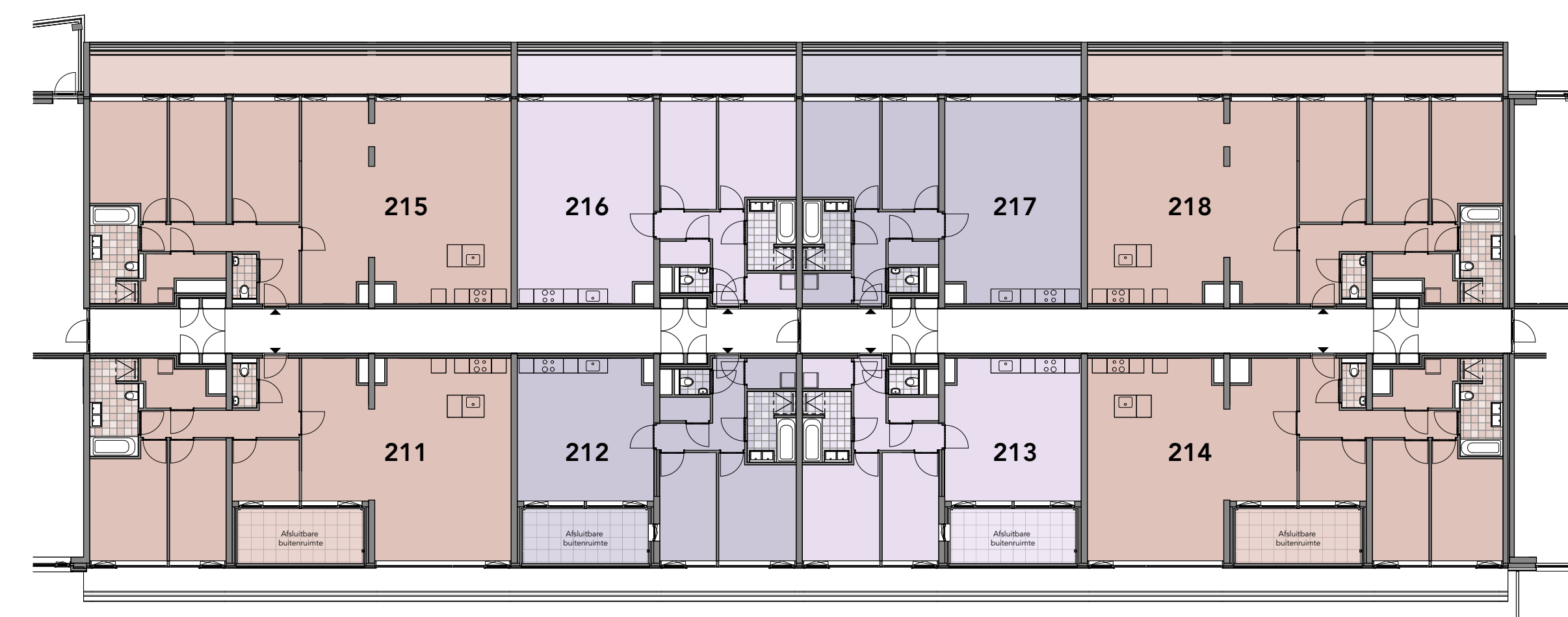
3e verdieping
