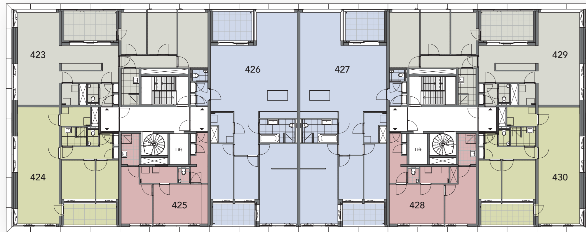
Derde verdieping
