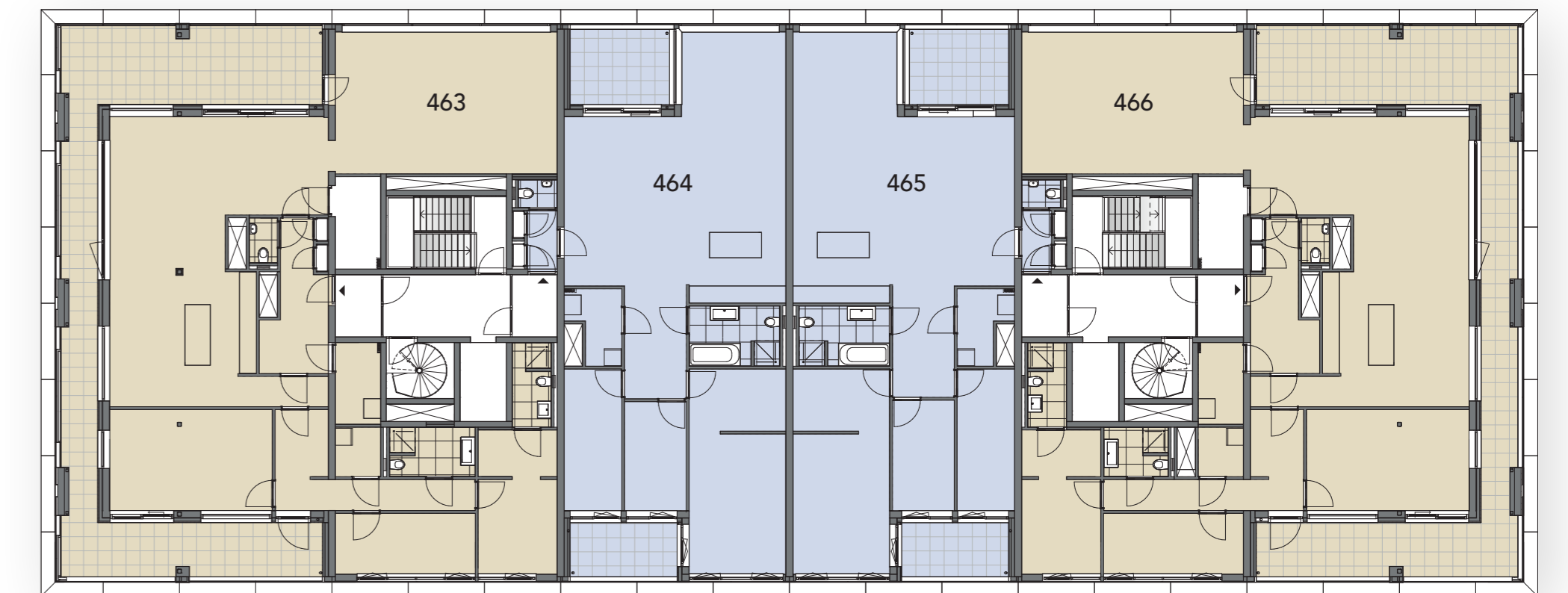
Achtste verdieping
