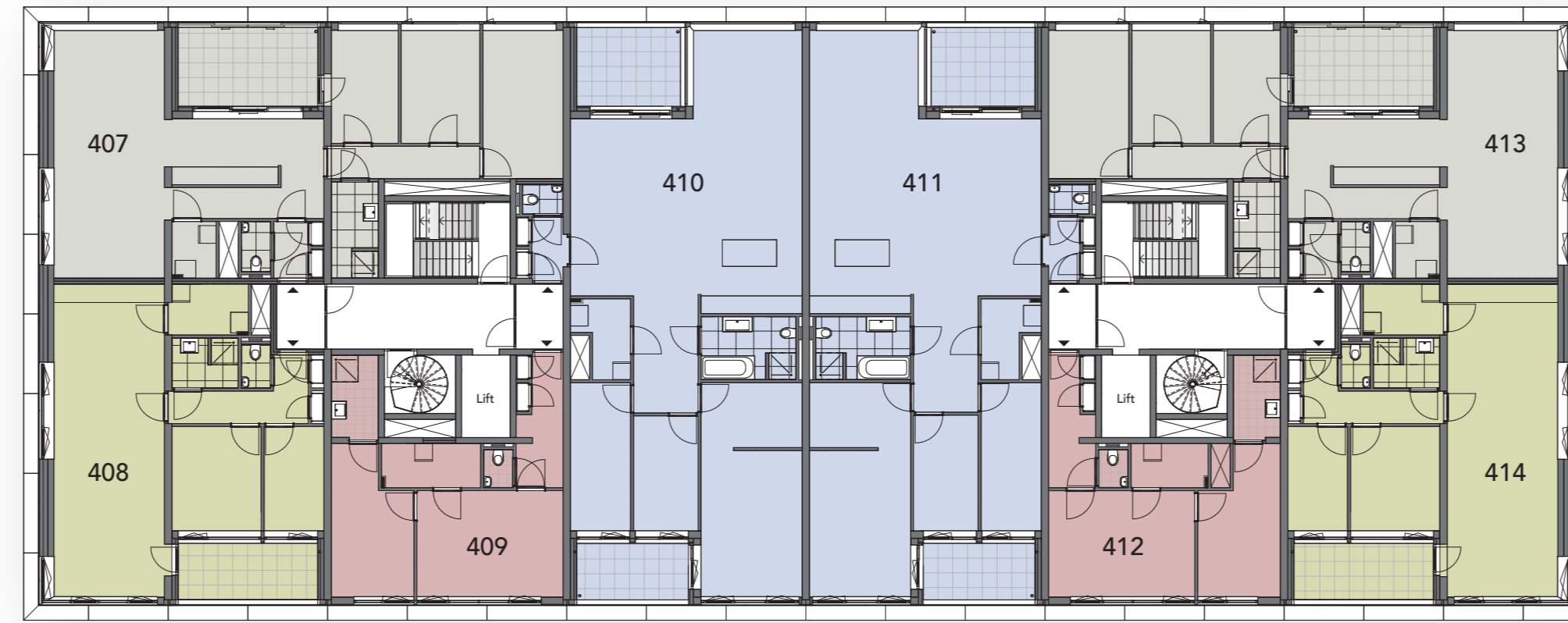
Eerste verdieping
