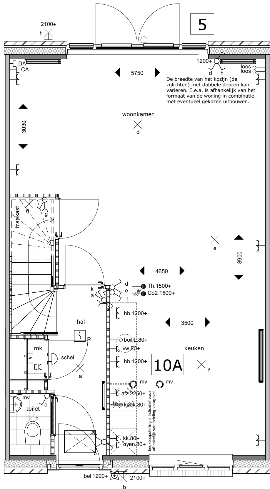
beuk 6000mm dubbele deur (optie 5) rechte keuken (optie 10A)
