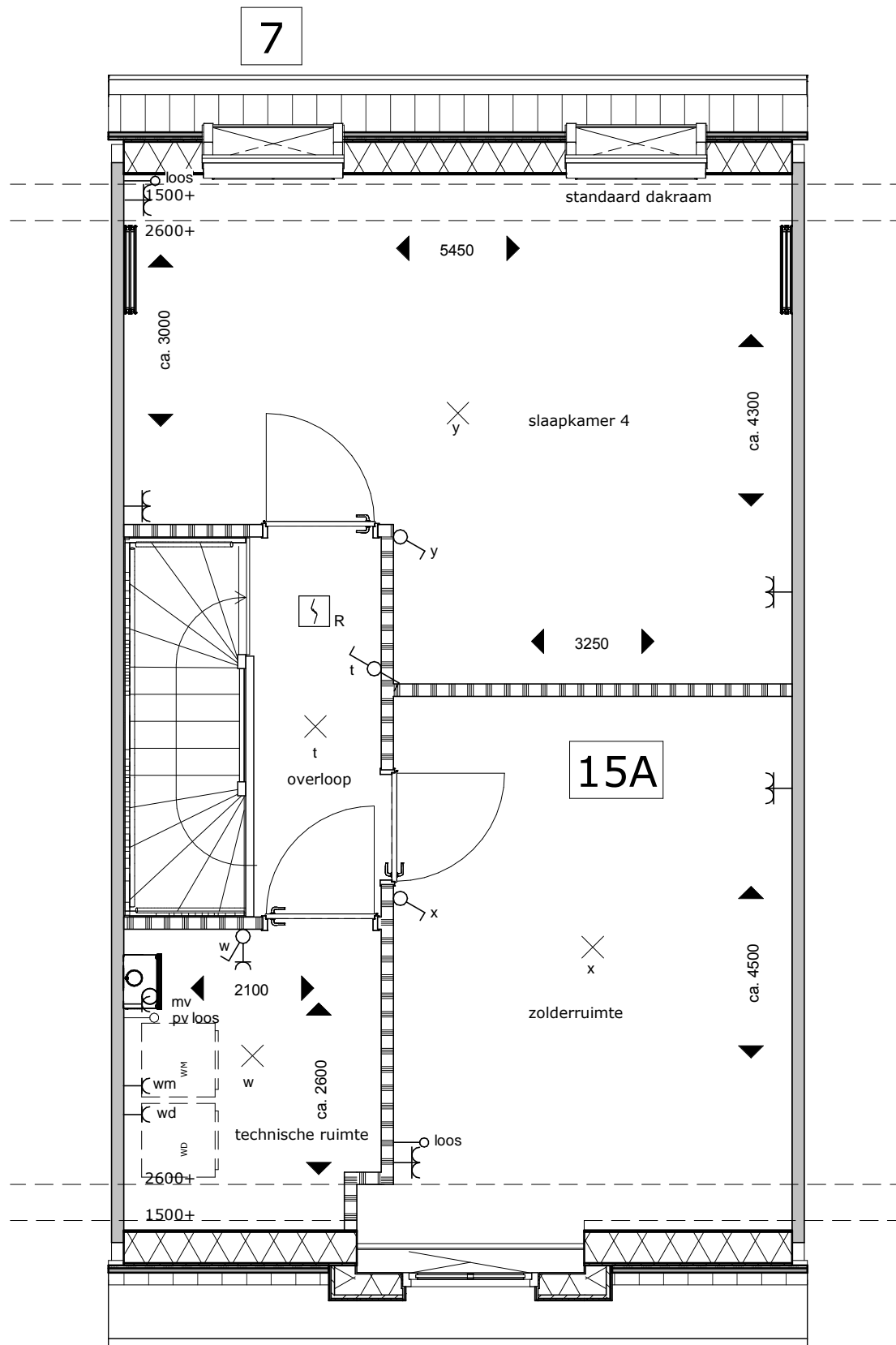
beuk 5700mm extra dakraam (optie 7) indelingsvariant 1 zolder (optie 15A)
