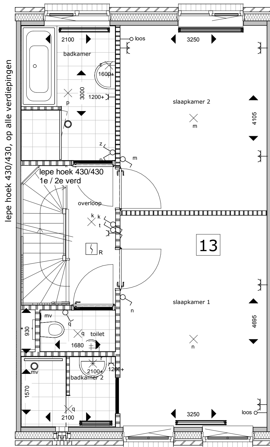
beuk 5700mm lifestyle variant 1e verd (optie 13)
