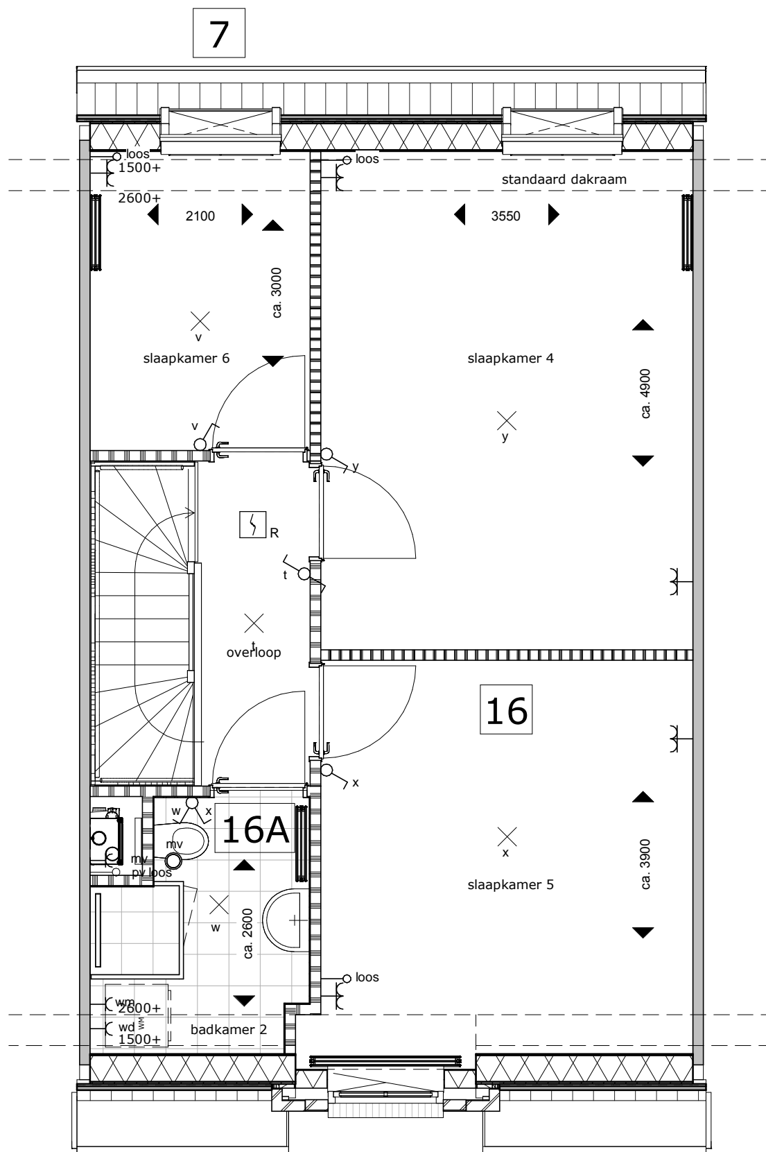
beuk 6000mm extra dakraam (optie 7) indelingsvariant 2 zolder met badkamer (optie 16+16A)
