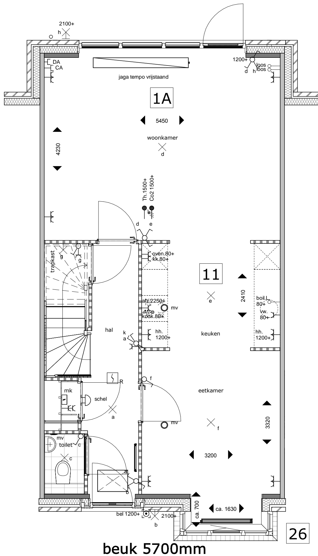
beuk 5700mm lifestyle variant 1 bgg (optie 11) i.c.m. uitbouw 1200 (optie 1A), erker voorgevel (optie 26) en vergrote pui achtergevel.
