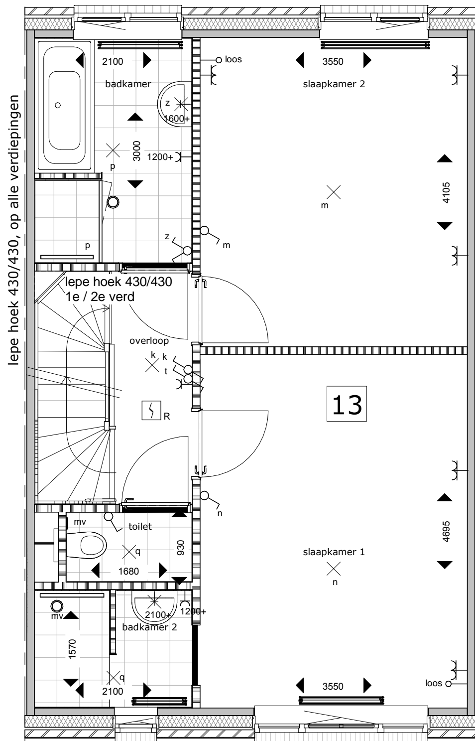
beuk 6000mm lifestyle variant 1e verd (optie 13)
