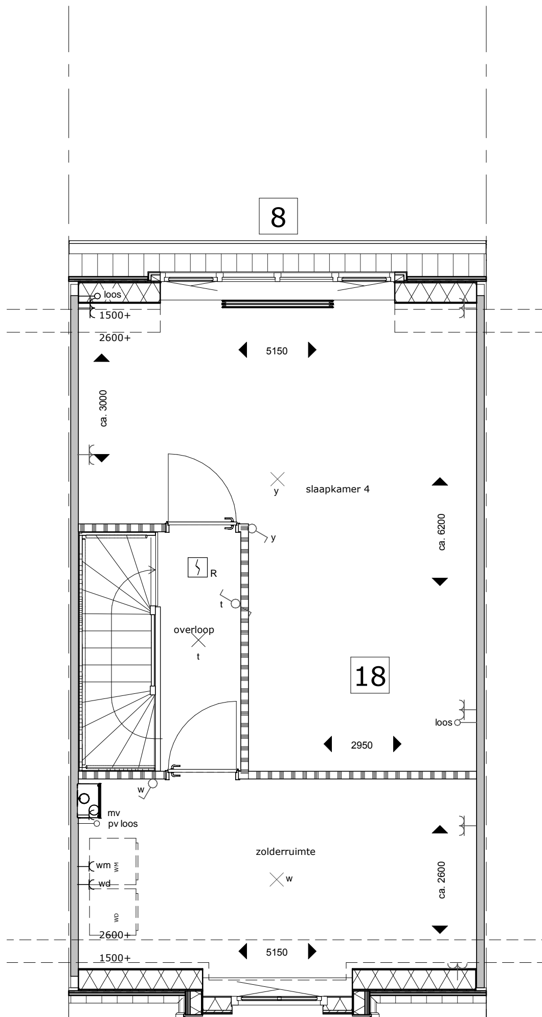
beuk 5400mm dakkapel achter (optie 8) indelingsvariant 4 zolder (optie 18)
