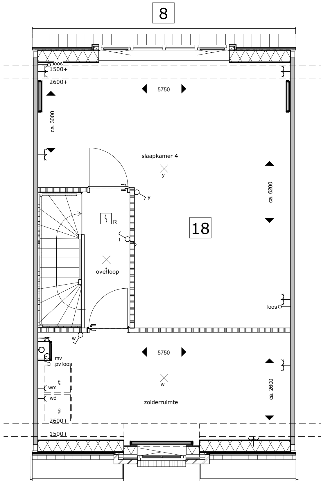
beuk 6000mm dakkapel achter (optie 8) indelingsvariant 4 zolder (optie 18)
