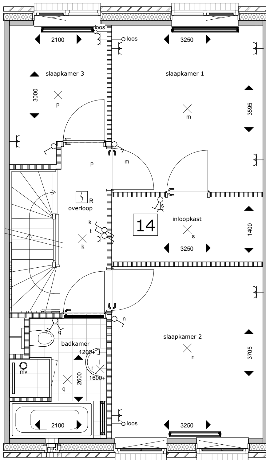
beuk 5700mm inloopkast (optie 14)
