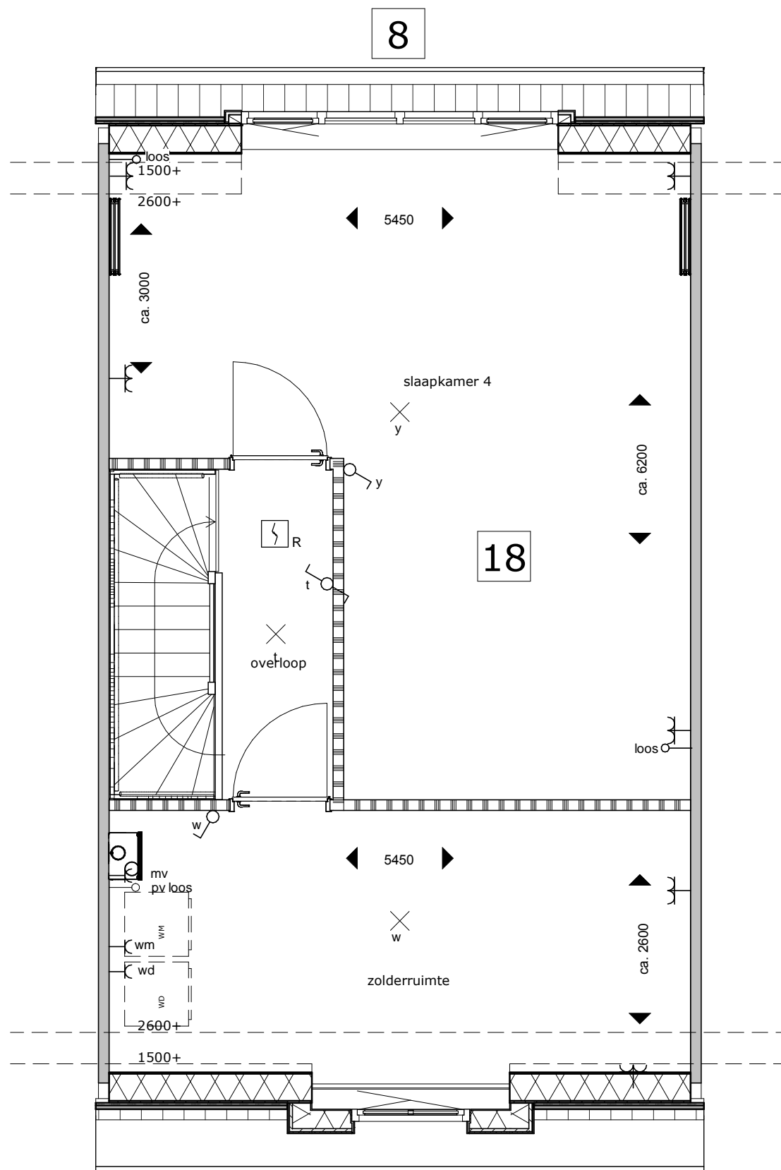
beuk 5700mm dakkapel achter (optie 8) indelingsvariant 4 zolder (optie 18)
