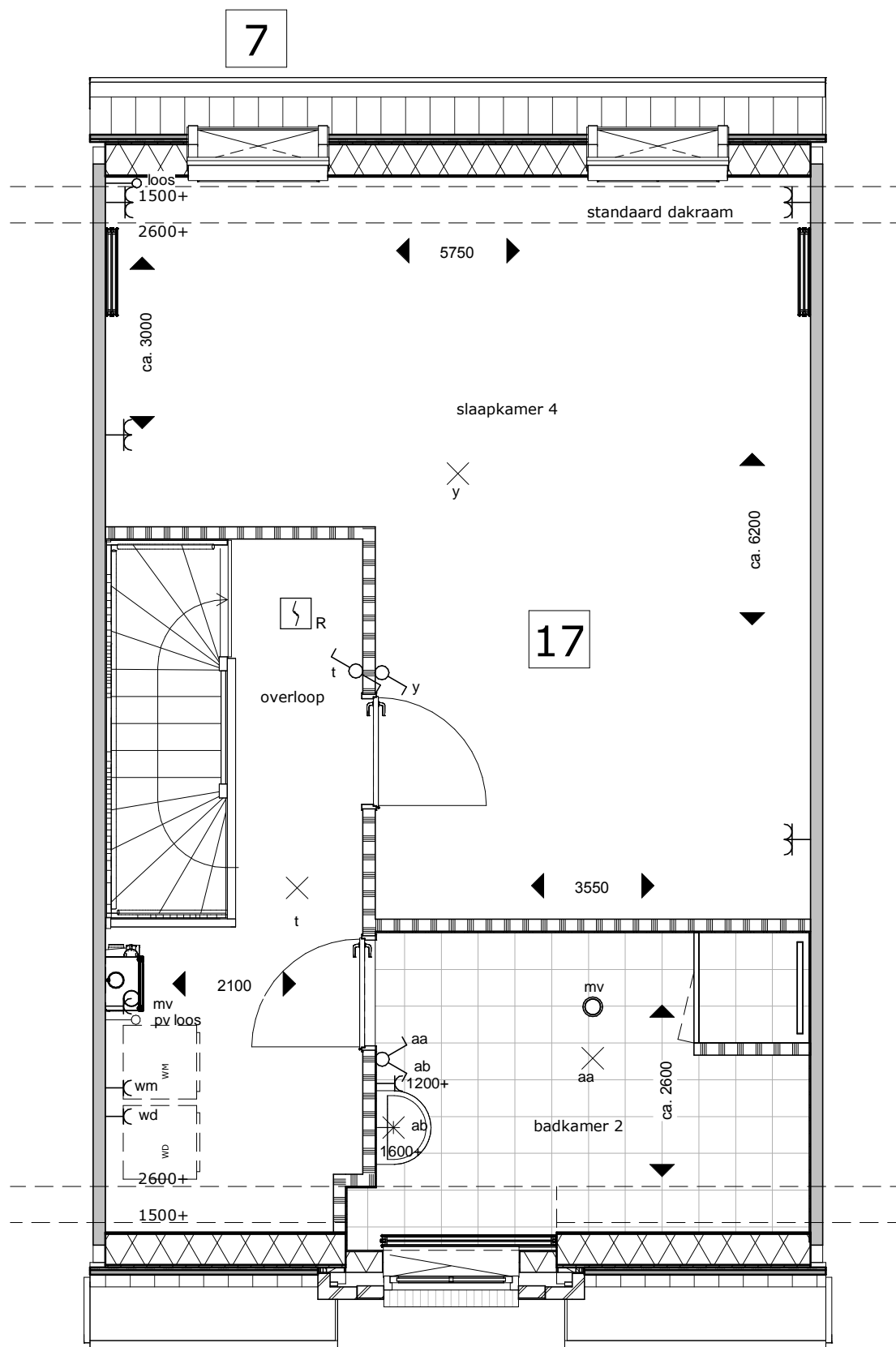
beuk 6000mm extra dakraam (optie 7) indelingsvariant 3 zolder met badkamer (optie 17)
