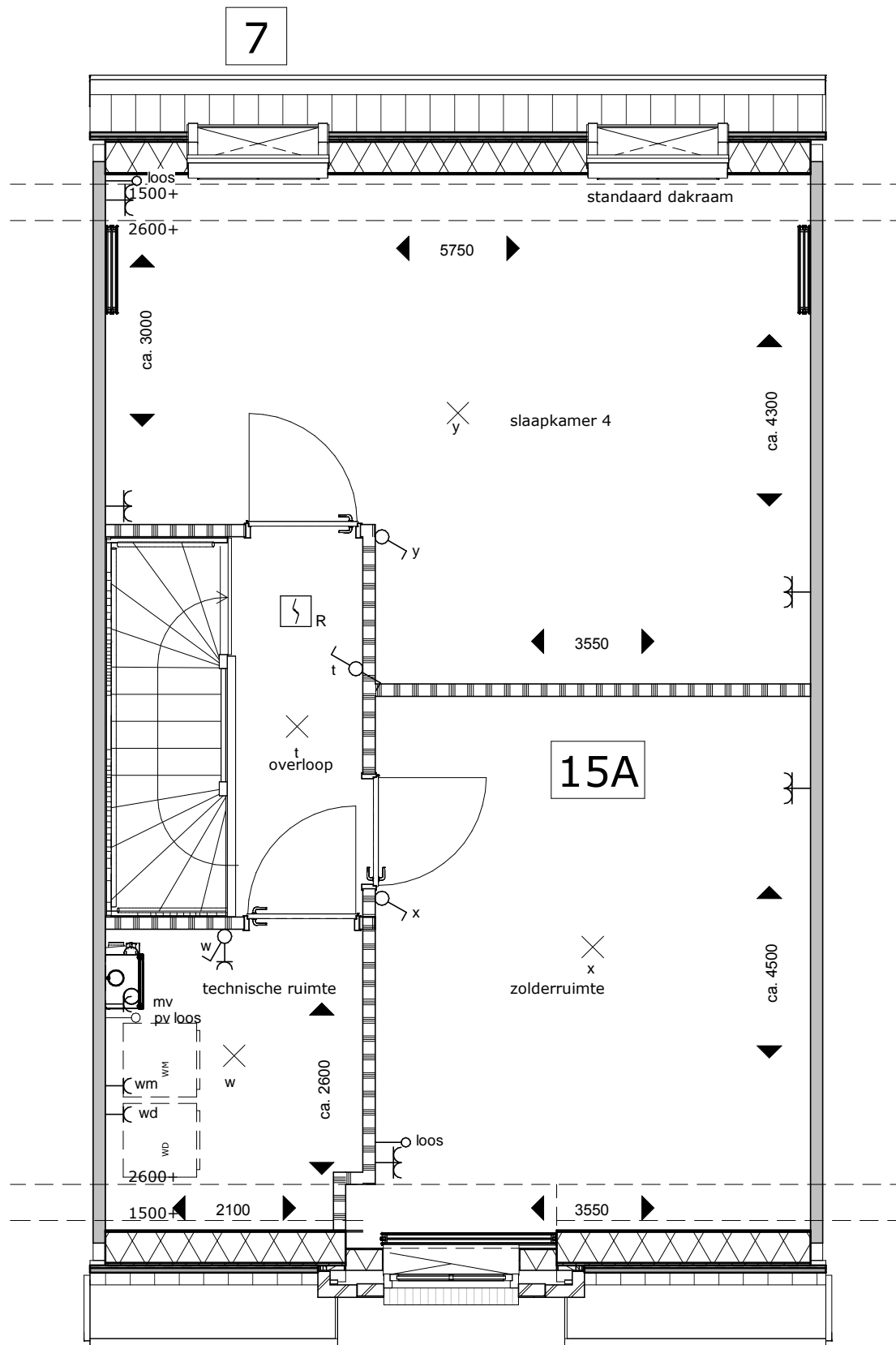
beuk 6000mm extra dakraam (optie 7) indelingsvariant 1 zolder (optie 15A)
