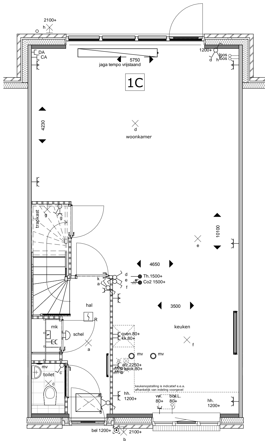
beuk 6000mm uitbouw 1200 (optie 1C) i.c.m. vergrote pui achtergevel
